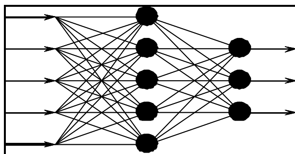
Рис. 5. Перцептрон (сеть с последовательными связями)
